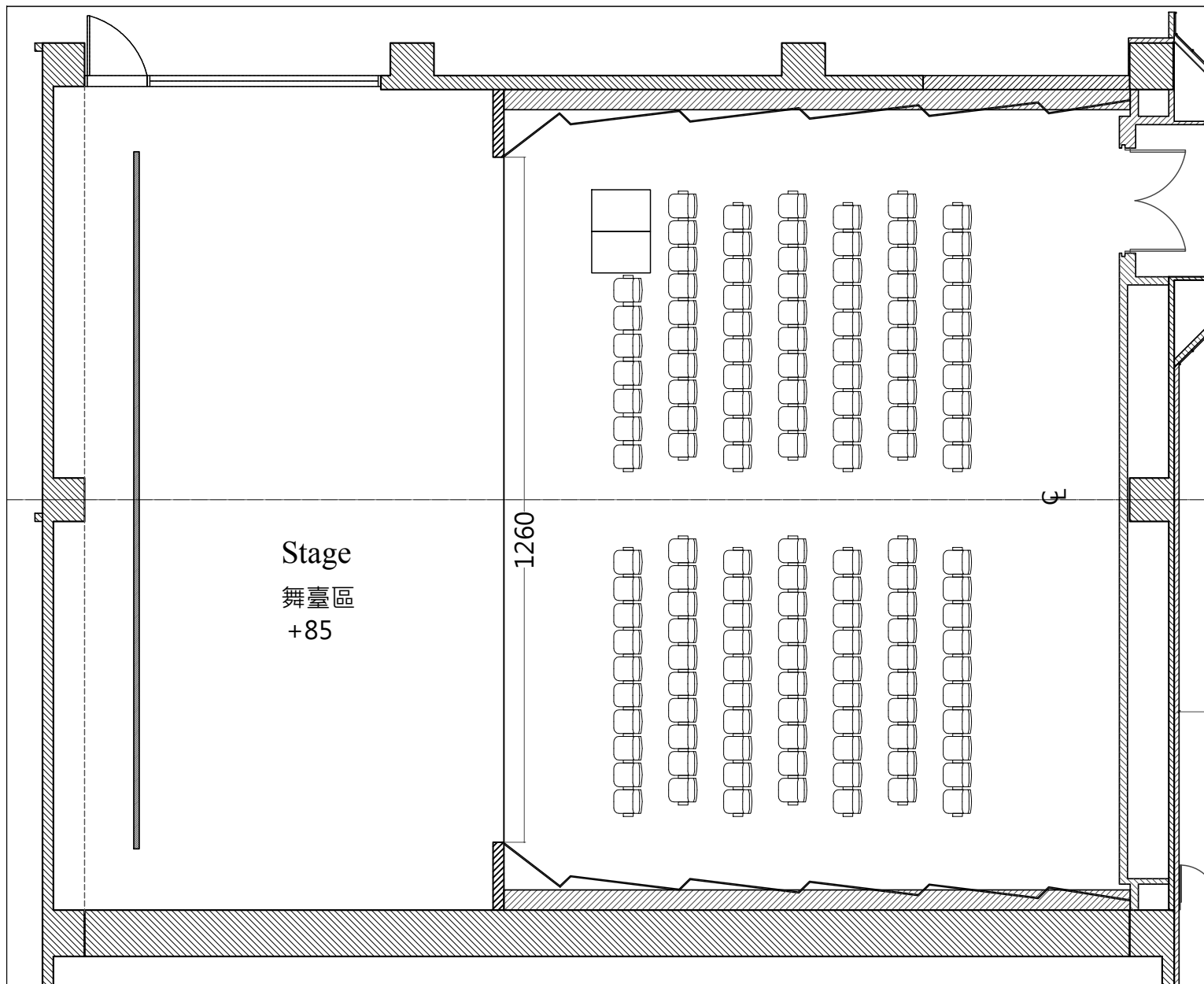
圖 (三) 小舞台(3201)_座位圖 (單位：公分) Figure(3) Small Stage(3201)_Auditorium Plan (Unit: cm)
