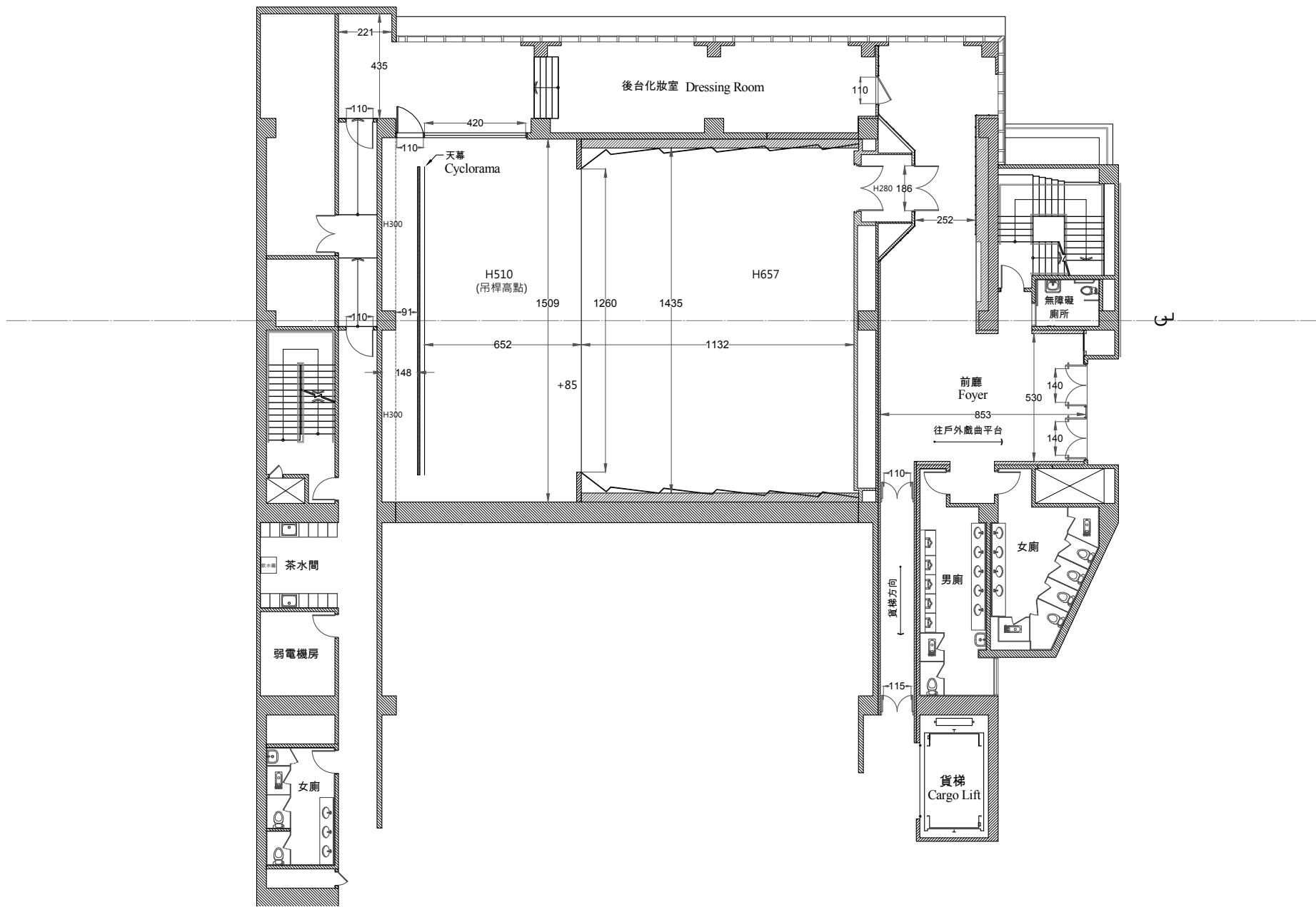
圖 (一) 小舞台(3201)_平面圖 (單位：公分) Figure(1) Small Stage(3201)_Floor Plan (Unit: cm)
